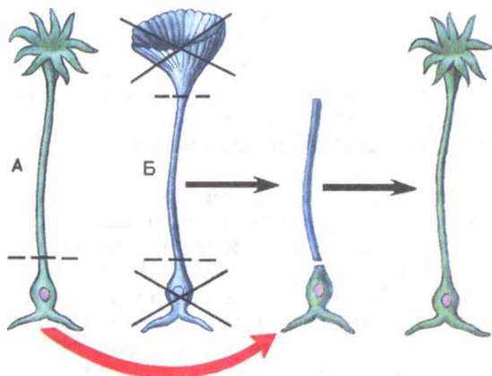
Рис. 18. Схема опыта с ацетабулярией. А и Б — разные виды ацетабулярий
