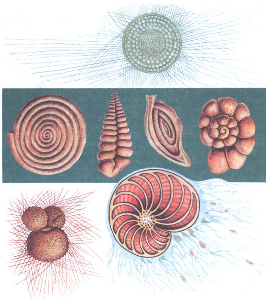
Рис. 79. Фораминиферы. Вверху и внизу — живые формы; посередине — скелеты вымерших форм, образующих мел
