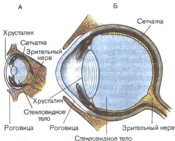
Рис. 64. Пример схождения в строении глаз. А — строение глаза головоногого моллюска — каракатицы; Б — строение глаза млекопитающего
