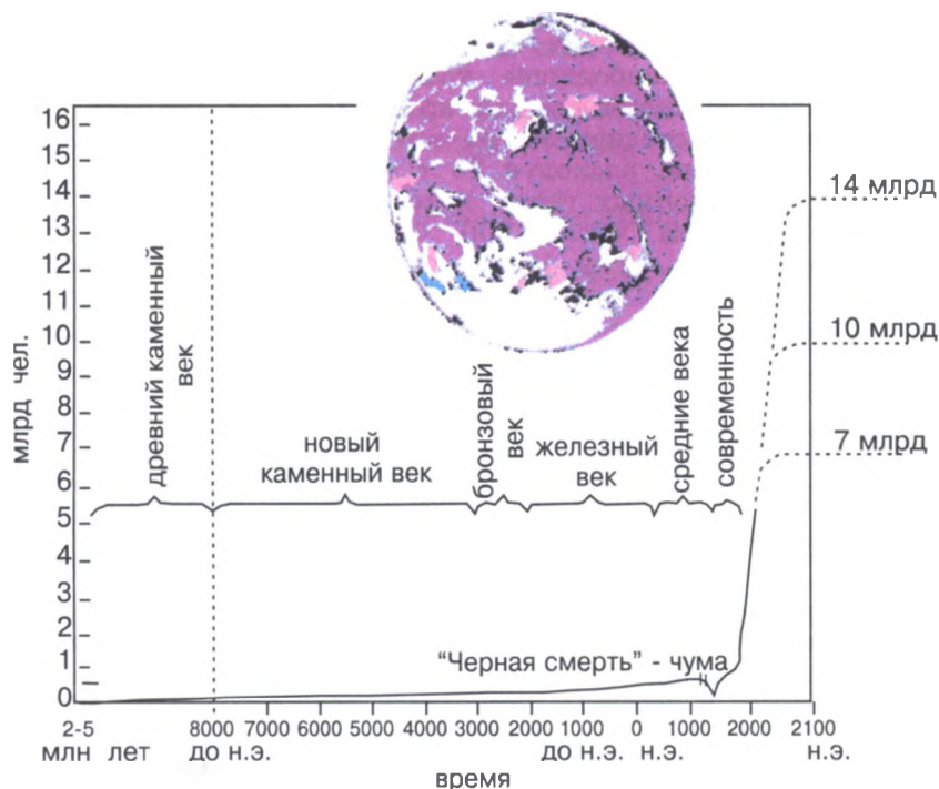
Рис. 110. График экспоненциального роста численности населения в прошлом и прогнозе на 2100 г.
