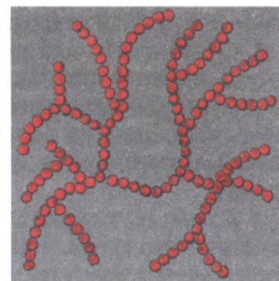
Рис. 3. Участок ветвящейся полимерной молекулы крахмала, где каждое звено — глюкоза
