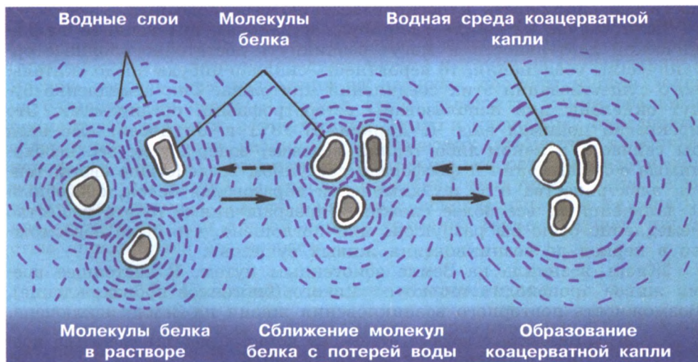
Рис. 70. Образование коацерватной капли
