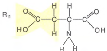
Аспарагиновая кислота (асп)
