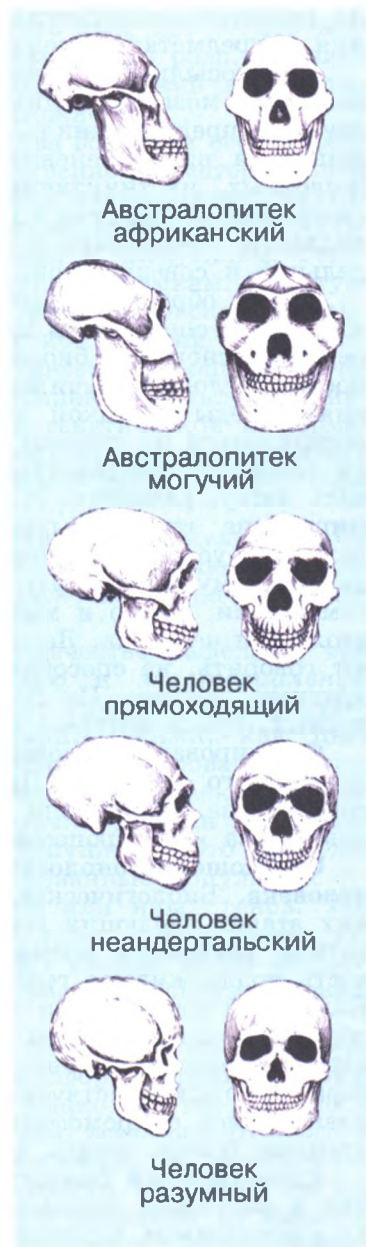
Рис. 101. Изменение пропорций черепа в ходе эволюции гомининов
