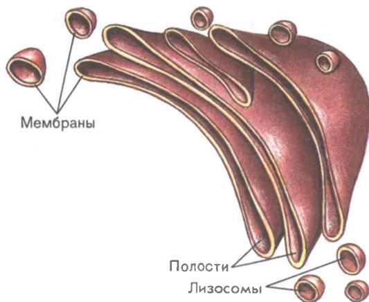
Рис. 14. Схема строения комплекса Гольджи
