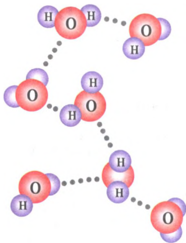
Рис. 1. Образование водородных связей в воде
